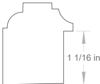
A&M # 60155 1-3/8" X 1-5/8"
